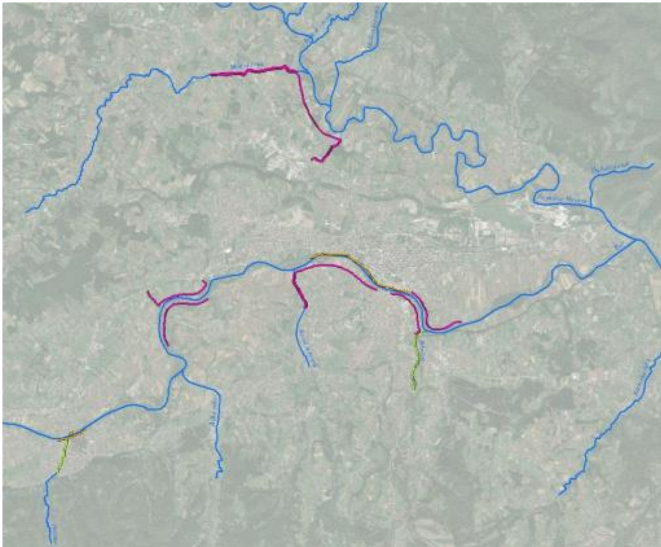
Слика – Систем одбране од поплава на територији града Краљева (преузето из - Мапирање области погодних за инсталацију мобилних система одбране од поплава на сливу реке Западне Мораве, извор: https://riskzm.rs/wp-content/uploads/2021/10/MAPIRANJE_PP_SISTEMI_GIR_2021.pdf )
