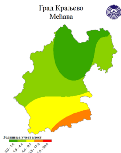
Просторна расподела учесталости међаве за Град Краљево
