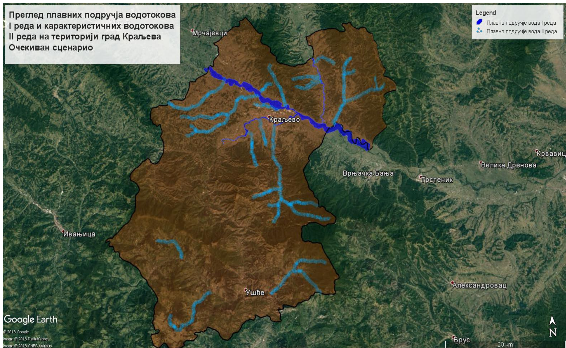
Слика број 3. – Преглед плавних подручја водотокова I реда и карактеристичних водотока II реда на територији града Краљево
