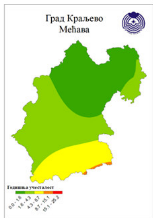
Просторна расподела учесталости међаве за Град Краљево
