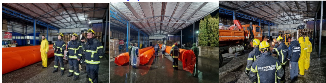
Фотографије 1-3 – инсталација мобилних противпоплавних система на локацији Екофарм Ушће код Краљева, јануар 2023. год. (извор: Цивилна заштита Краљево)
