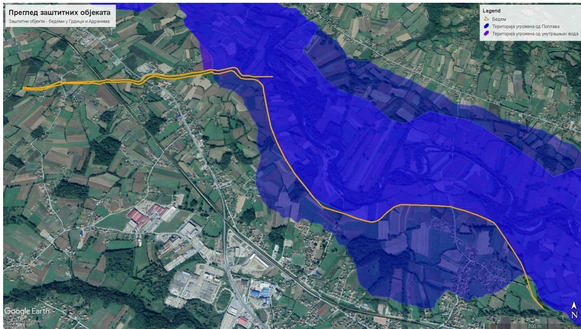
Слика број 6. – Преглед заштитних објеката на водама I реда
