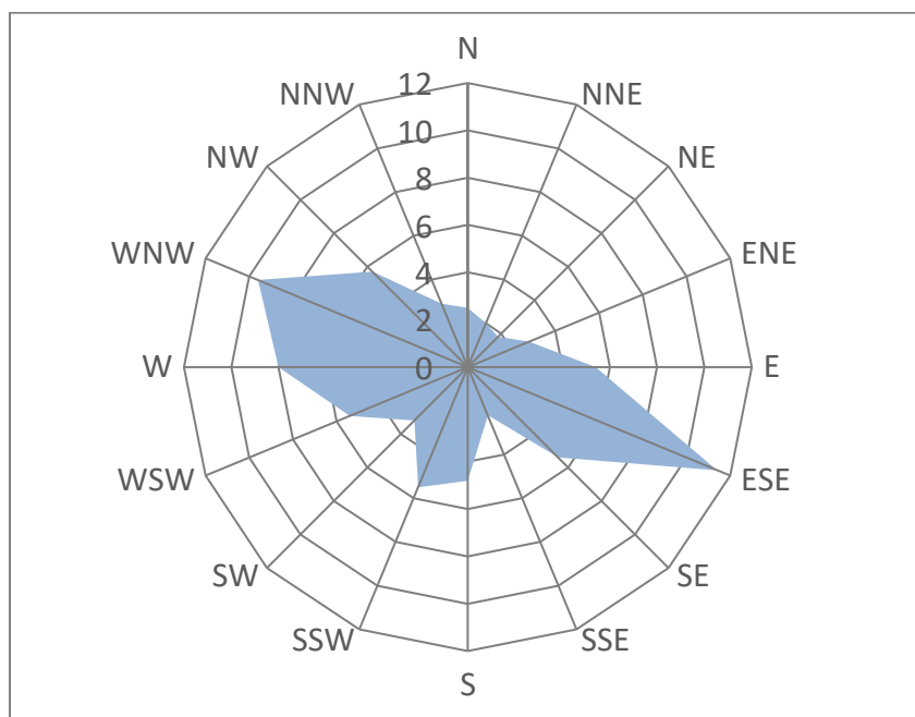
Слика Error! No text of specified style in document.-2 Ружа ветрова за климатолошки период 1991-2020
